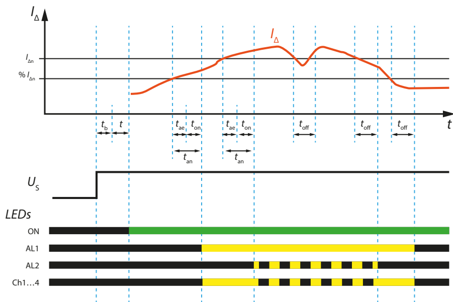
Abbildung 2-1: Zeitdiagramm
