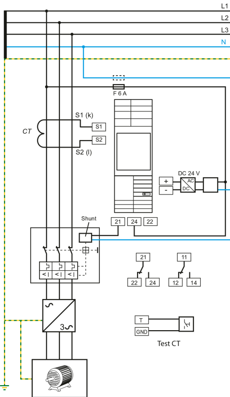
Anschlussbild Shunt-Auslöser
